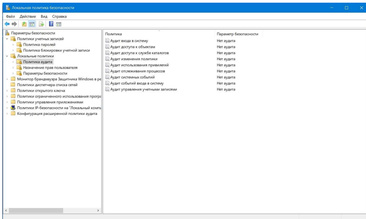
Рисунок 17 – “Политика аудита”.
