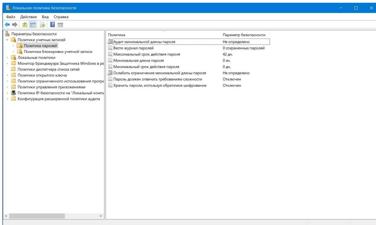
Рисунок 15 – “Политика настроек”.
