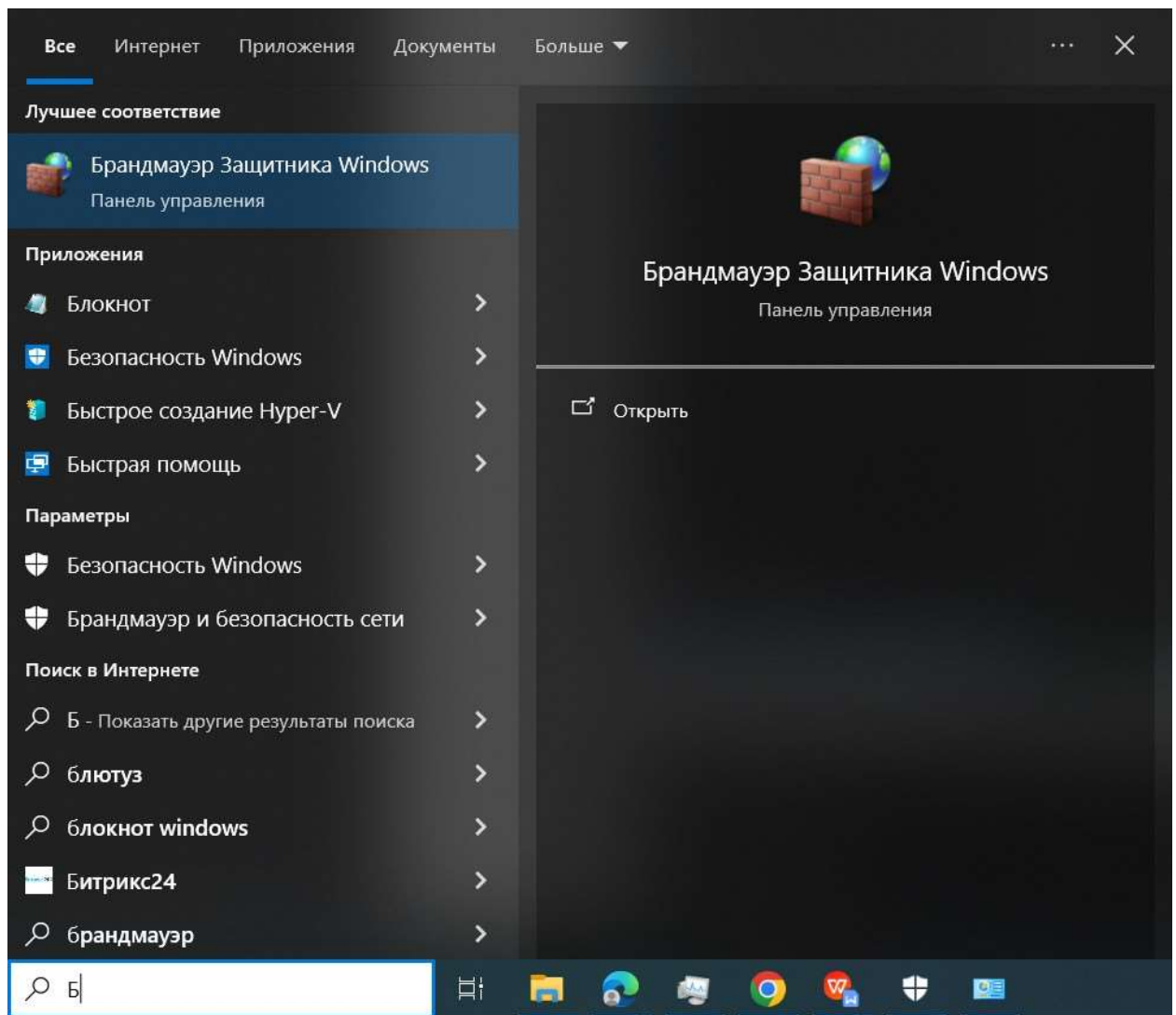
Рисунок 8 – Меню “Пуск”.
