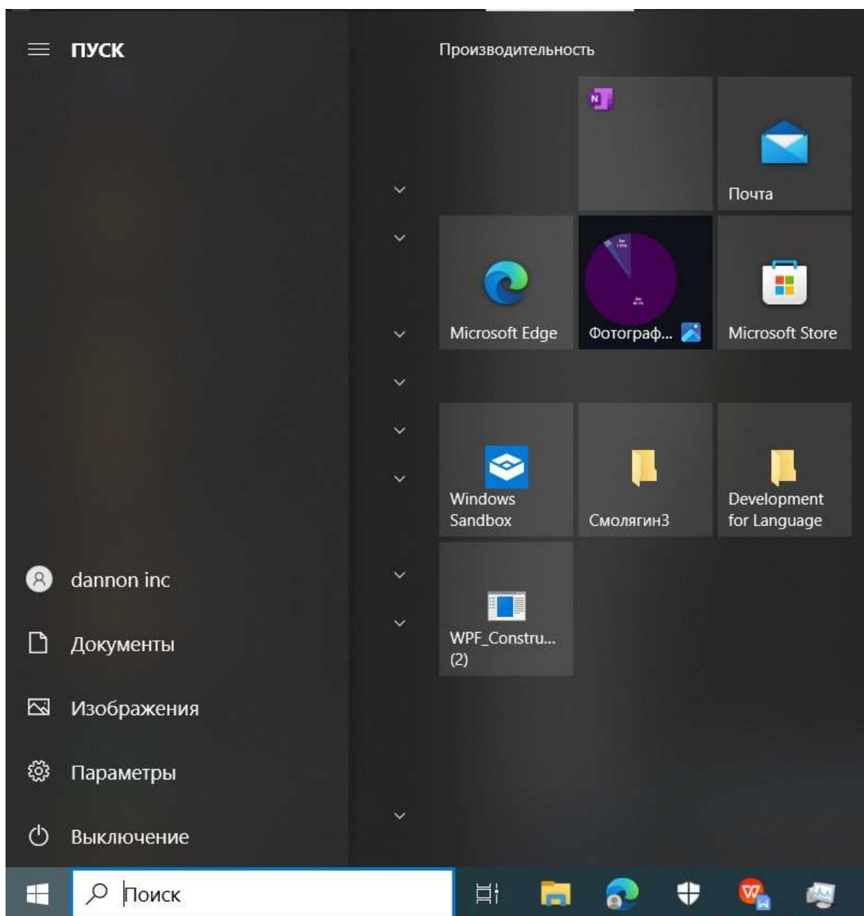
Рисунок 1 – Меню “Пуск”.
